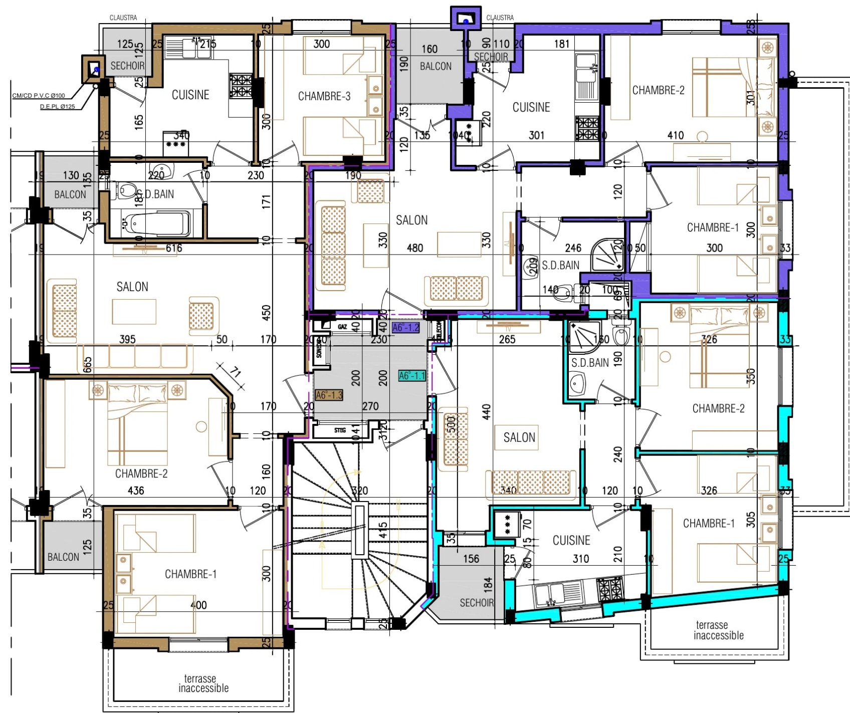
PLAN 1er ETAGE
