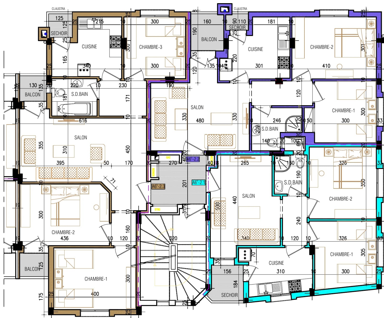
PLAN 2eme ETAGE
