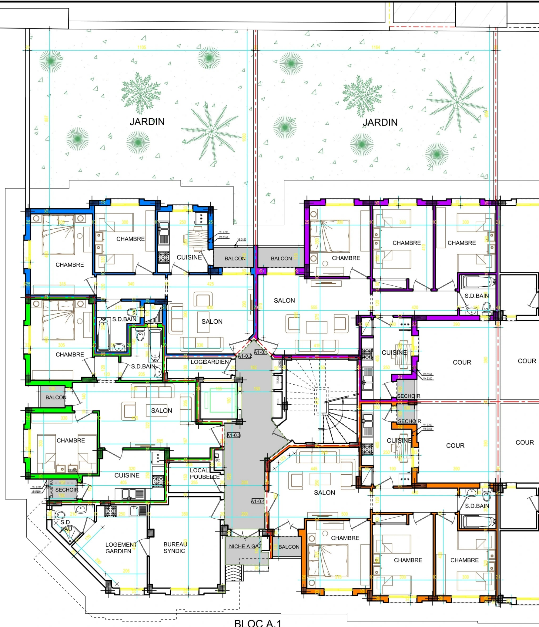
PLAN REZ-DE-CHAUSSEE
